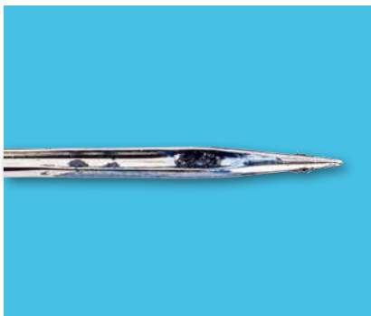
粘附着残留物的标准机针
